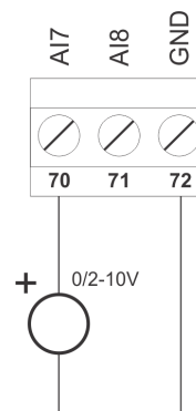
Figura 2.3 – Ligação para sensores saída tensão.
