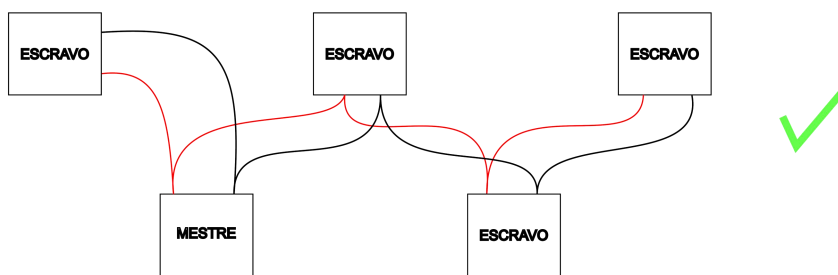
Figura 9 - Ligação encadeada ( Daisy Chain ).
