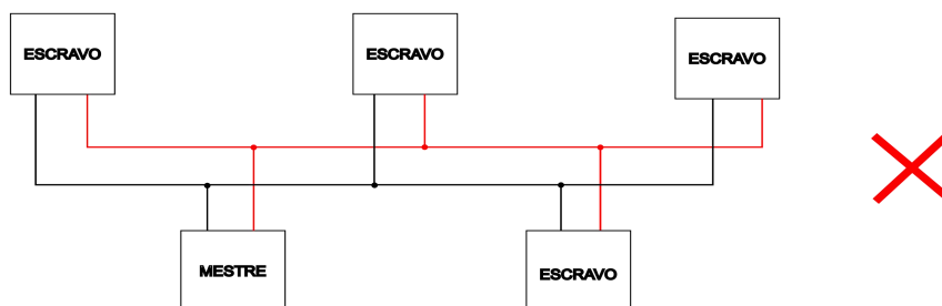
Figura 10 - Ligação em "T".
