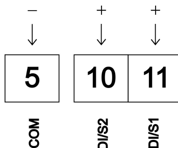
Figura 11 - Conexão das entradas digitais / NTC.
