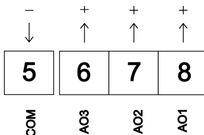
Figura 14 - Conexão das saídas analógicas.
